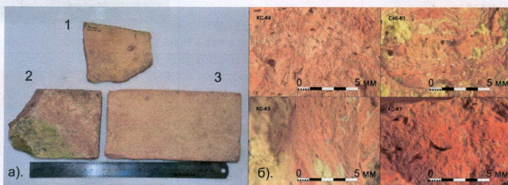
Рис. 2. а) Строительные элементы крепостей Сочи и Севастополис.
