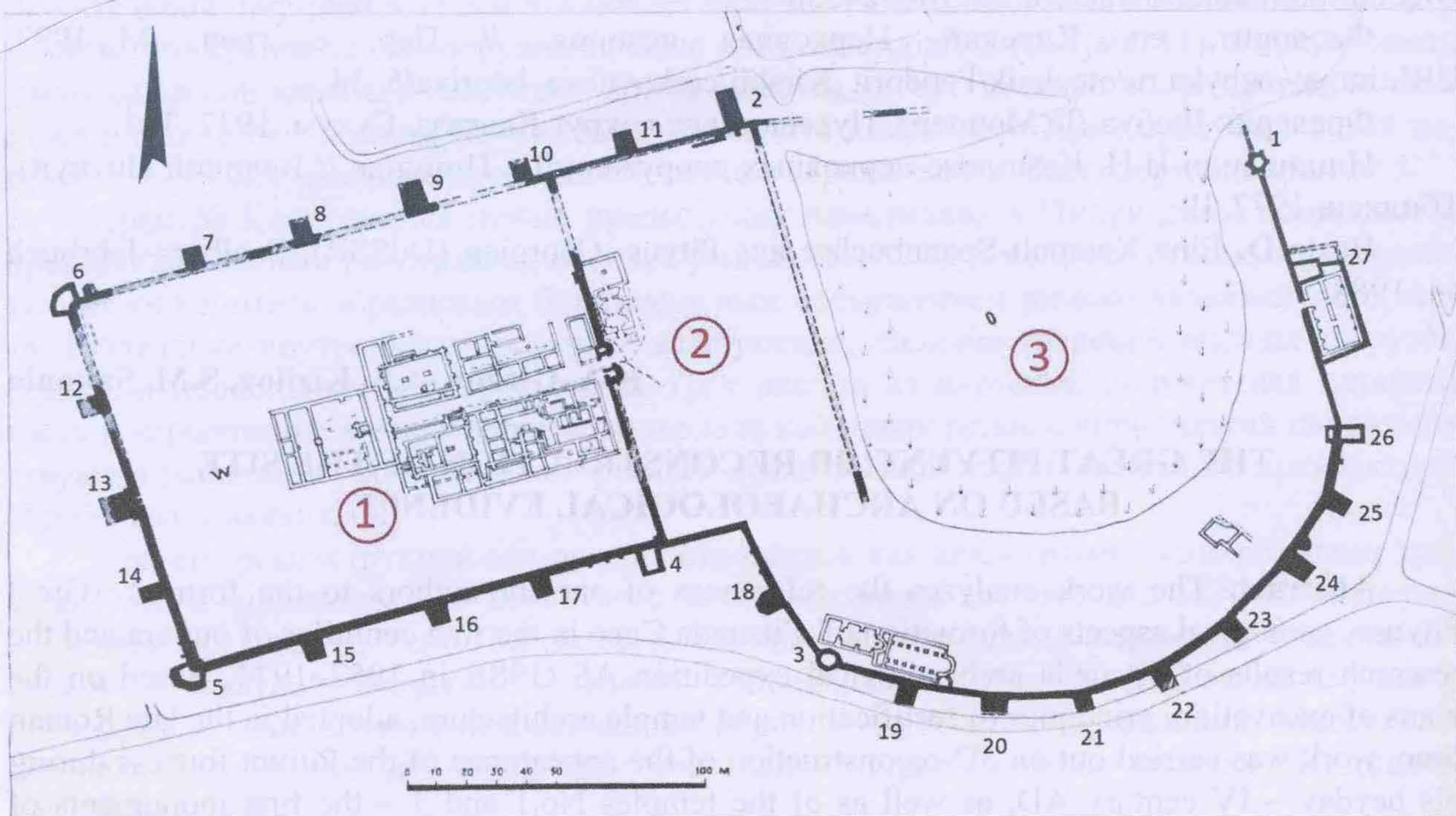
Рис. 2. Генеральный план Питиунтской крепости: 1 – кастеллум (конец II – начало III вв. н.э.); 2 – расширение кастеллума на восток (середина III в. н.э.); 3 – канаба (конец III – середина IV вв. н.э.).
