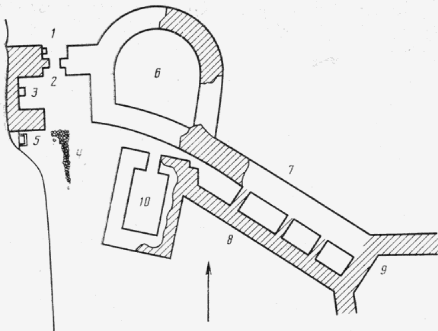
Рис. 2. План укреплений Ванского городища: 1 — катаракта; 2 — калитка; 3 — приватное сооружение с алтарем; 4 — мостовая; 5 — жертвенник; 6 — полукруглая башня; 7 — оборонительная стена (первая линия); 8 — оборонительная стена (вторая линия); 9 — многогранная башня; 10 — казарма.
